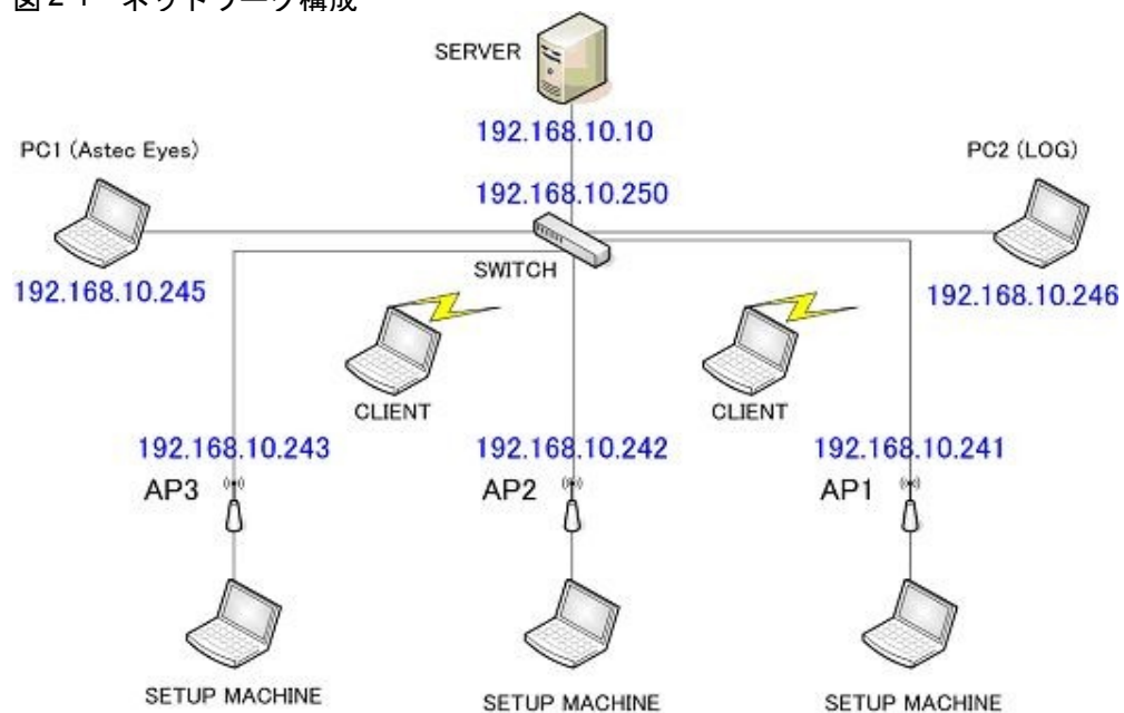
図 2-1 ネットワーク構成
